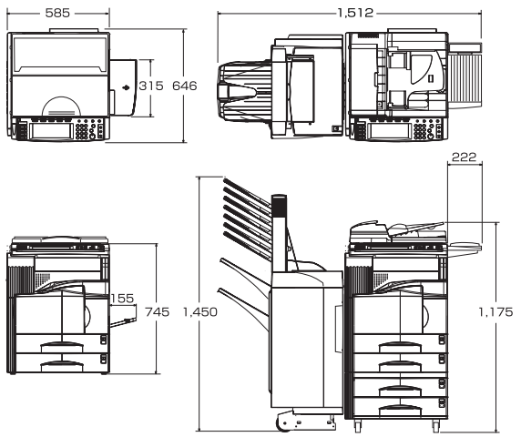
KM-4035の外形寸法 単位:mm
